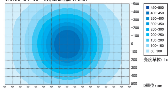
CWA3S-24-CD（測量距離：1m）
