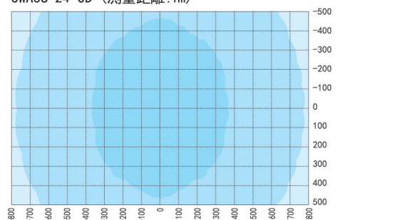
CWA3S-24-CD（測量距離：1m）
